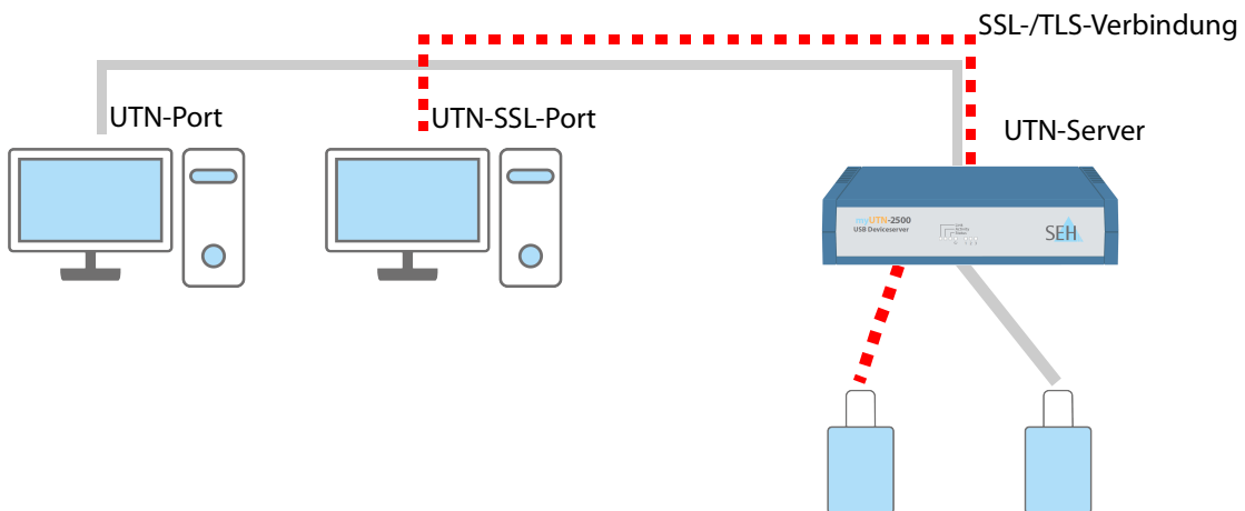
Abbildung 7: UTN-Server – SSL-/TLS-Verbindung im Netzwerk
