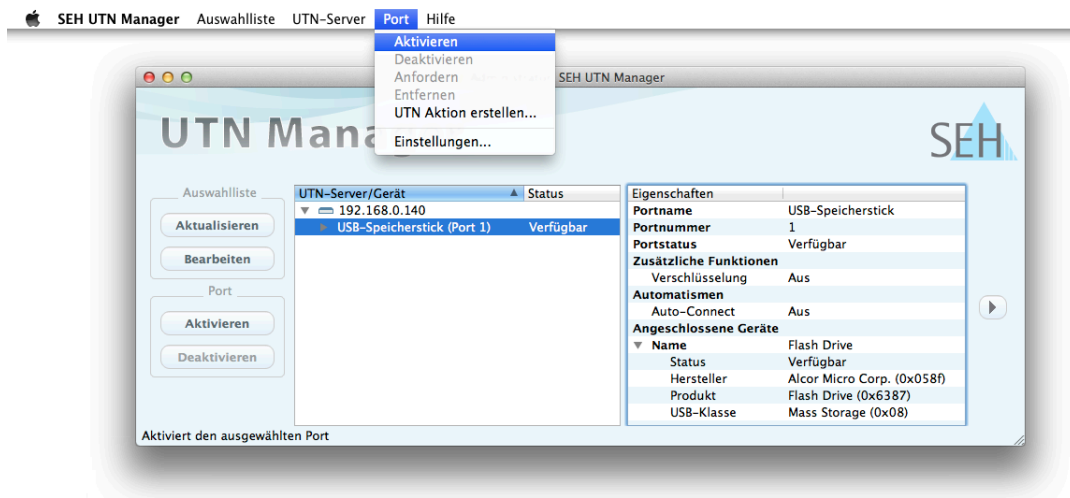
Abbildung 5: SEH UTN Manager – USB-Port aktivieren
